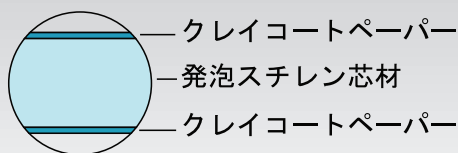
FOME-COR® 断面図
